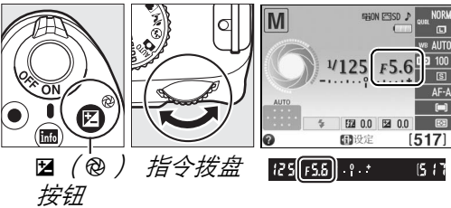
光圈
